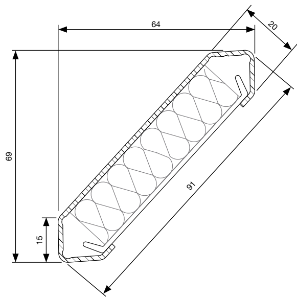
Doorsnedetekening
