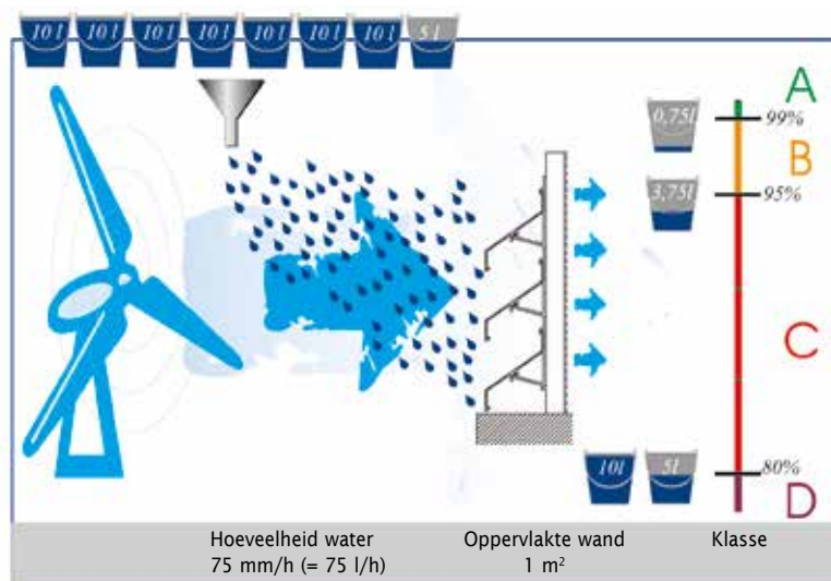
Test van een standaard lamellenwandsysteem
