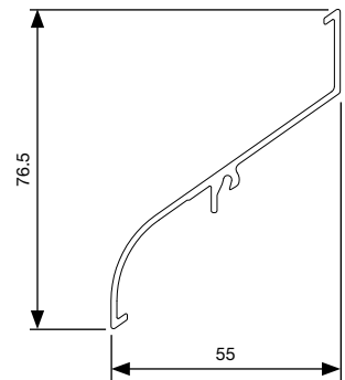
L.066S - projectprofiel
