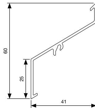
L.050.25 - projectprofiel
