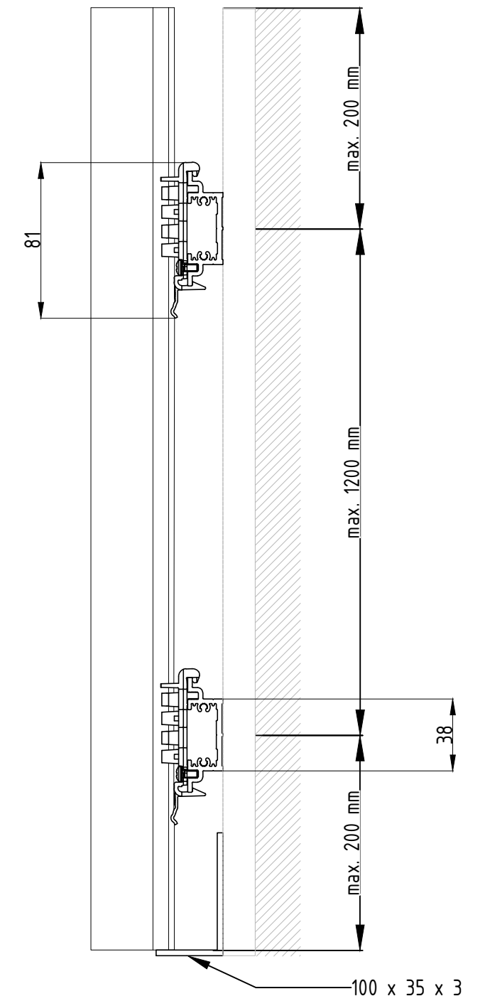
Doorsnede A-A
