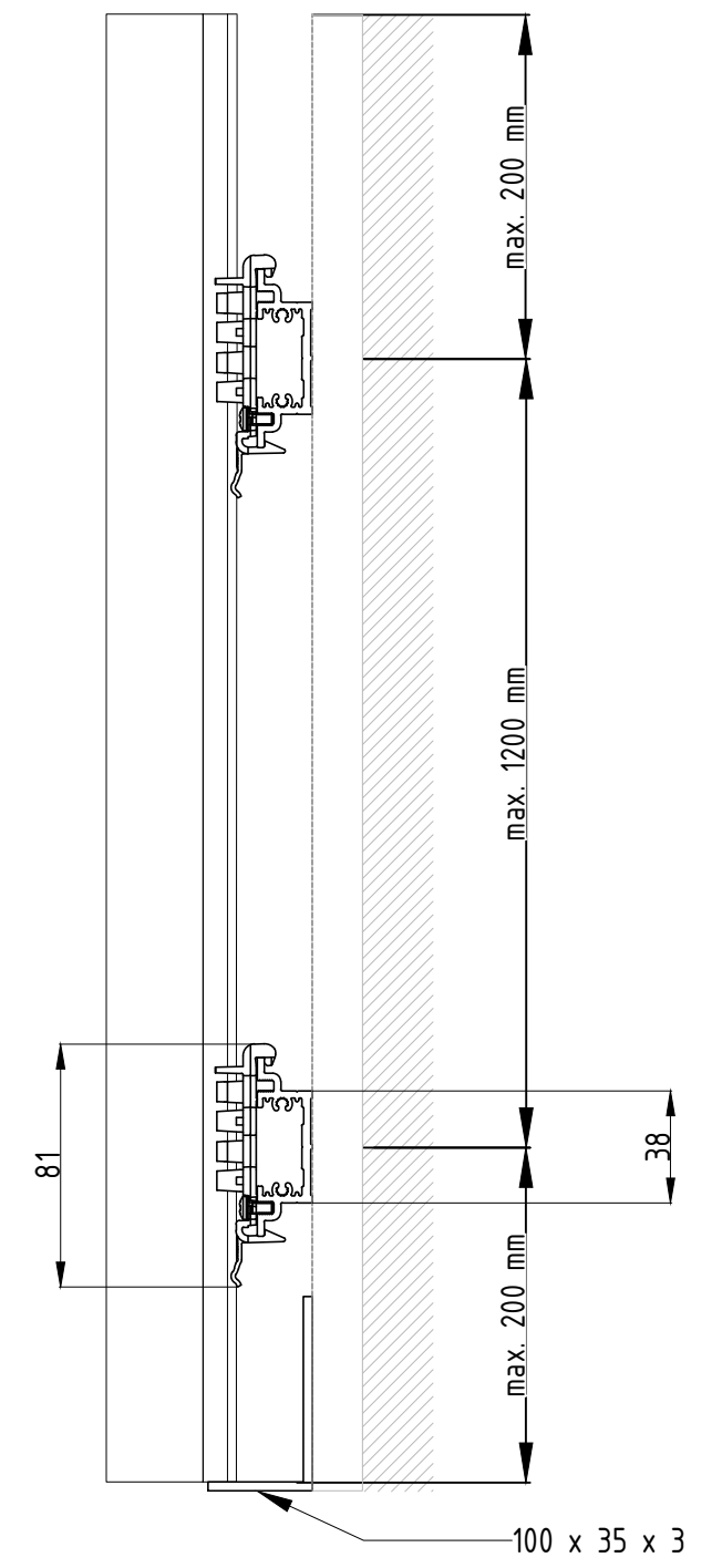
Doorsnede A-A
