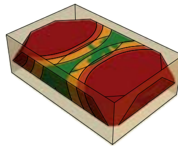
Warmte effect met 2 zijden verwarmd (formaat 6 x 4 m)
