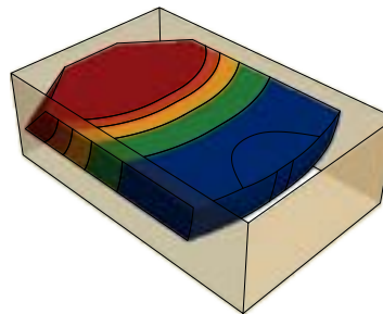
Warmte effect met 1 zijde verwarmd (formaat 6 x 4 m)
