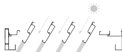
Direct zonlicht
