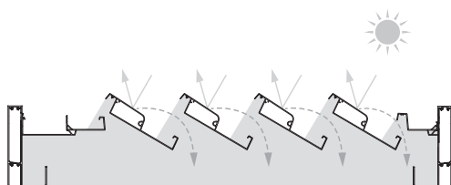
Indirect zonlicht
