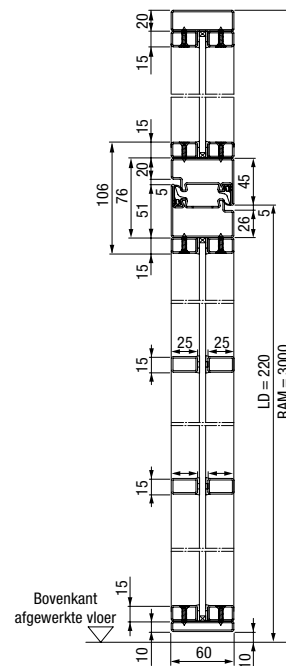
Verticale doorsnede 2-vleugelige stalen loftdeur met bovenlicht
