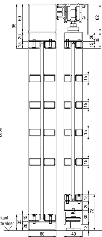
Verticale doorsnede 2-vleugelige stalen loftdeur met zijdelen
