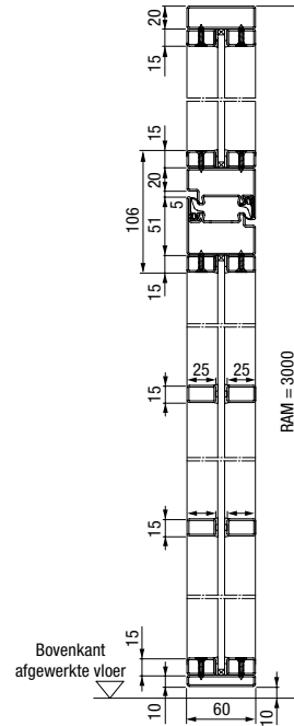
Verticale doorsnede 1-vleugelige stalen loftdeur met bovenlicht
