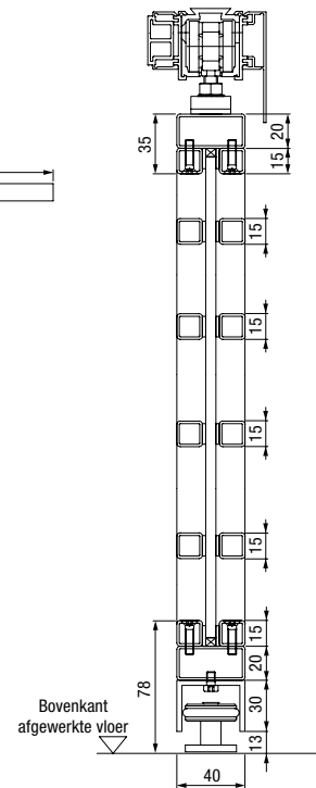
Verticale doorsnede 2-vleugelige stalen loftdeur
