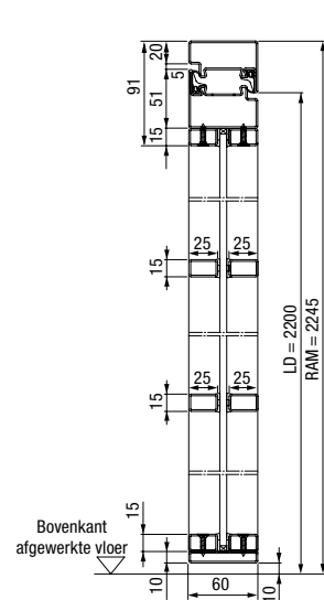
Verticale doorsnede 1-vleugelige stalen loftdeur
