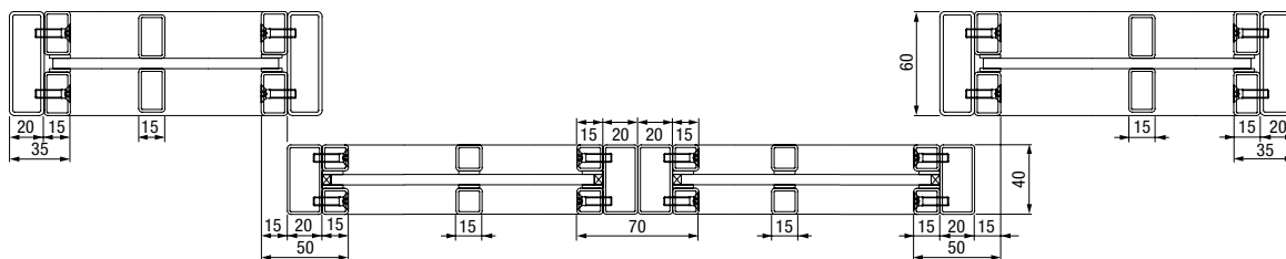
Horizontale doorsnede 2-vleugelige stalen loftdeur met zijdelen
