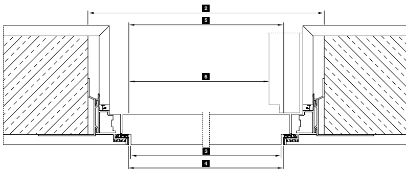
Zeroline – Breedte
