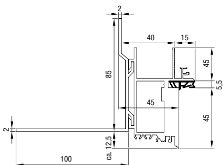
Maten Zeroline-kozijn
