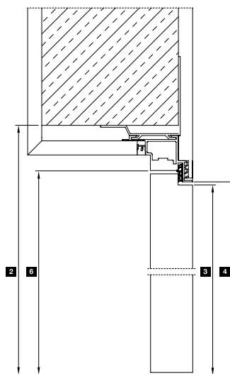
Verticale doorsnede reverse openend deurblad (met opdek)
