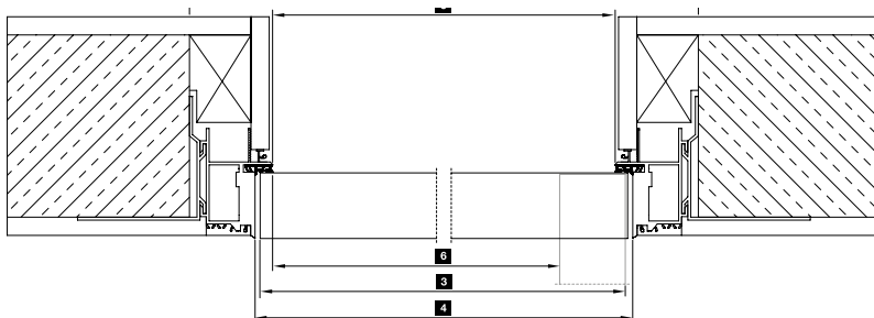
Horizontale doorsnede met stomp deurblad
