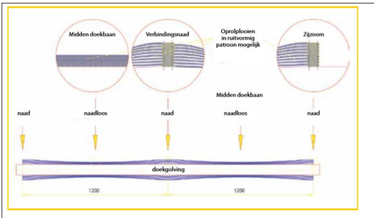
Afb. 9.1.11 Afwijkende roldiameter aan naden en zomen
