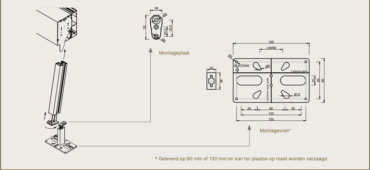
Bevestigingsmogelijkheden
