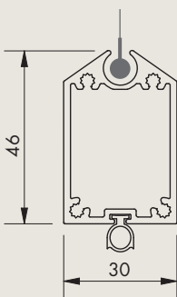
Onderlat
