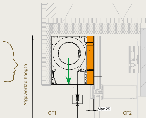
Verticale doorsnede - Reynaers Aluminium
