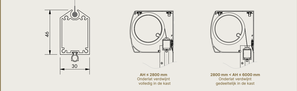
Fixscreen® 150 - Onderlat
