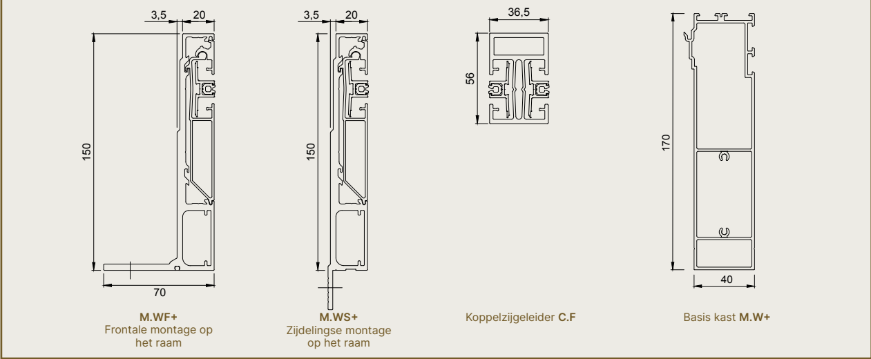
Montage met 40 mm uitvulling*
