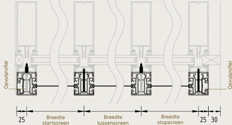
Horizontale doorsnede - Maatvoering
