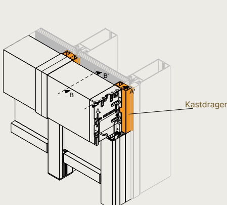
3D-aanzicht - Reynaers Aluminium
