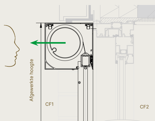
Fixscreen® 150 - Voorbouwtekening metselwerk
