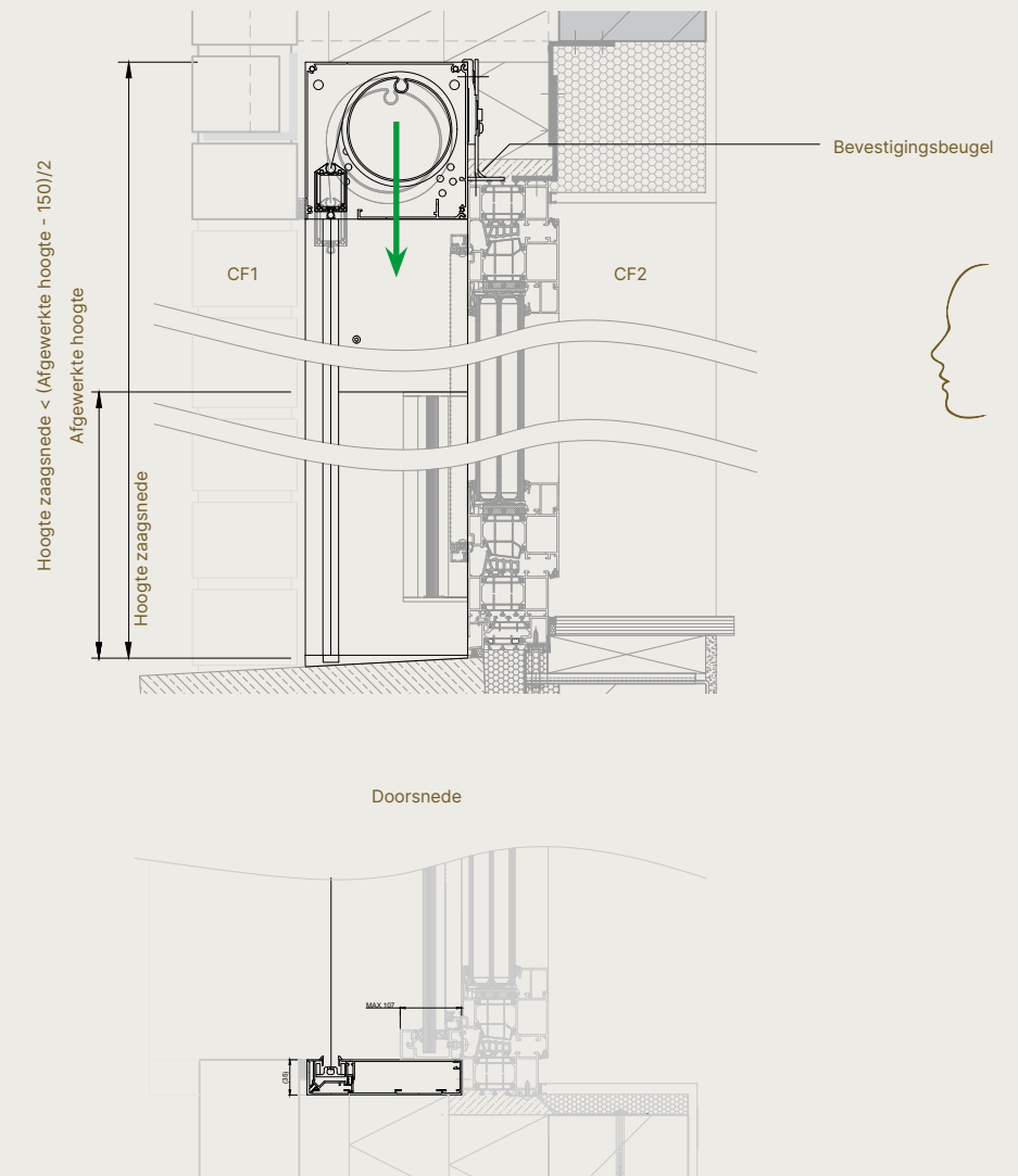
Fixscreen® 150 - MS 7B - Inbouwtekening balustrade
