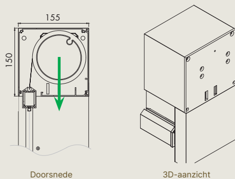
Fixscreen® 150 - MS 7B - Kast
