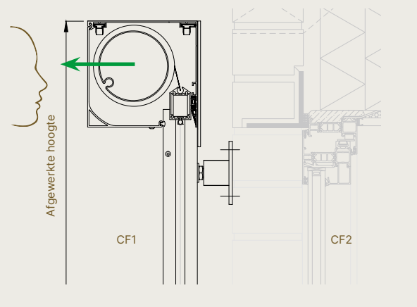
Fixscreen® 150 - Voorbouwtekening vliesgevel
