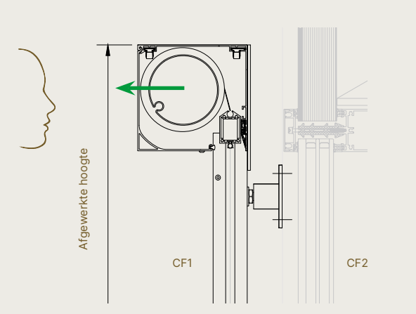
Fixscreen® 150 - Voorbouwtekening vliesgevel
