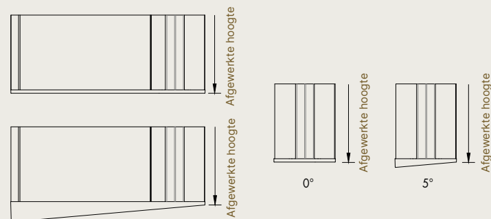
Voetplaat zijgeleider
