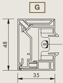
Fixscreen® 150 - Zijgeleiders
