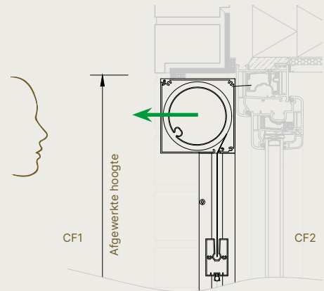
Fixscreen® 100 - Voorbouwtekening metselwerk
