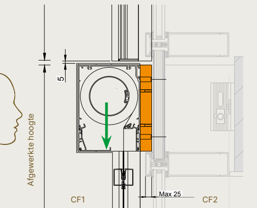
Verticale doorsnede doorlopende vliesgevel - Reynaers Aluminium
