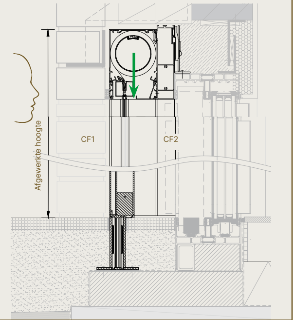
Medium - Metselwerk - MS 7B met C.F op montagevoet
