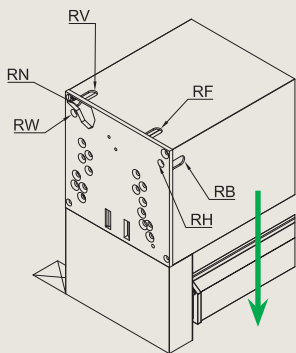
Kabeldoorvoer - MS 7B
