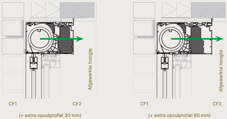
Voorbeeld 1: Medium op smaller raam
