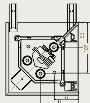
Hoekbeugel (positie boorgaten)
