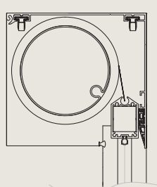
Fixscreen 150
