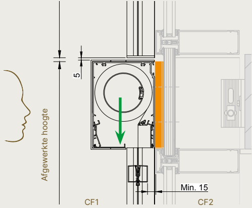
Verticale doorsnede doorlopende vliesgevel
