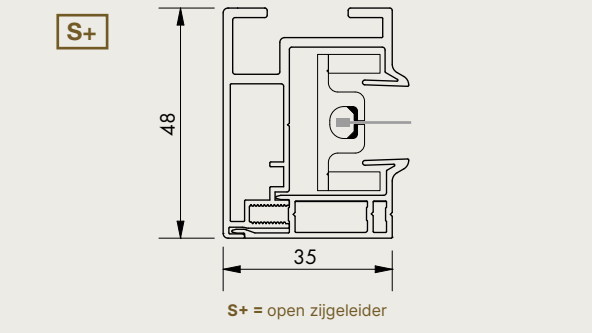
Zijgeleider
