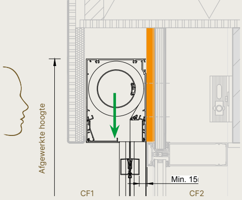
Verticale doorsnede
