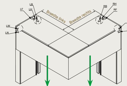
Kabeldoorvoer
