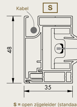
Zijgeleiders
