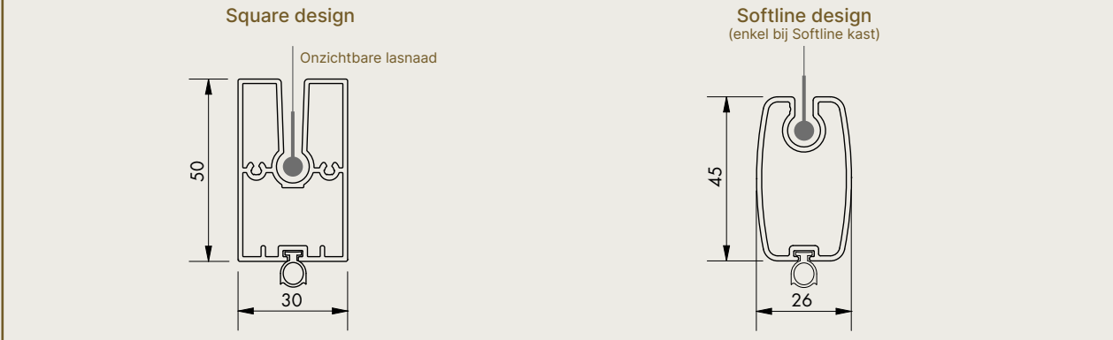
Fixscreen® 150 - Onderlat
