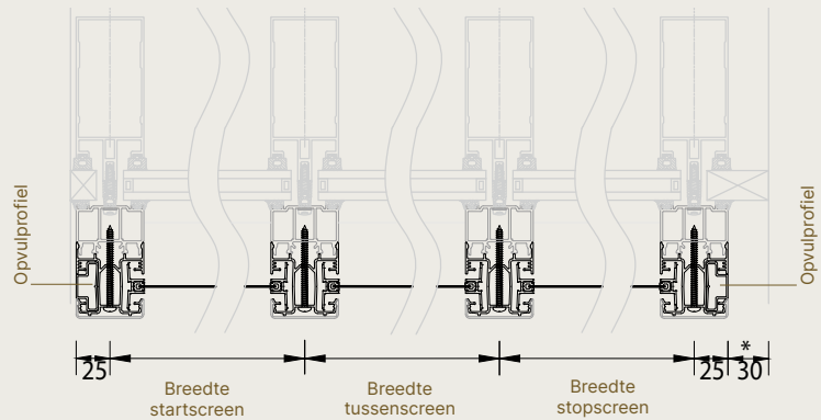
Horizontale doorsnede - Maatvoering - Reynaers Aluminium
