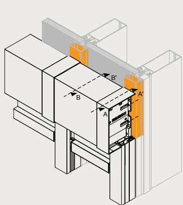
3D-aanzicht
