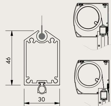
Fixscreen® 150 - Onderlat
