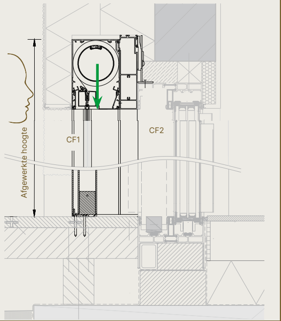
Medium - Pleisterwerk - MS 7B met C.F op montageplaat
