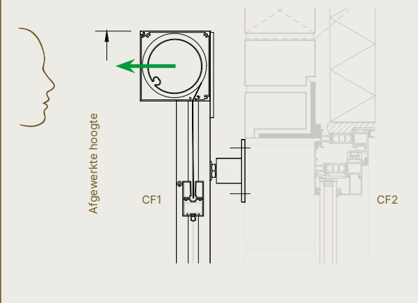
Fixscreen® 100 - Voorbouwtekening vliesgevel
