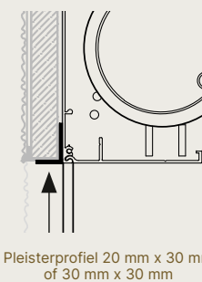
Pleisterprofiel
