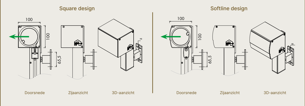
Fixscreen® 150 - Kast
