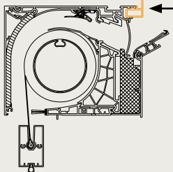
Afwerkingsprofiel (Optie)
