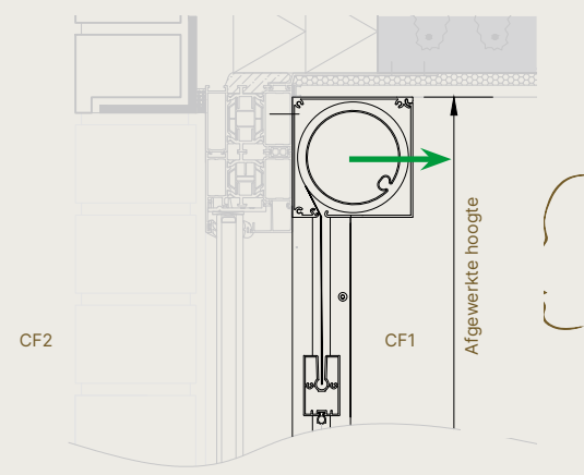
Fixscreen® 100 - Voorbouwtekening binnentoepassing
