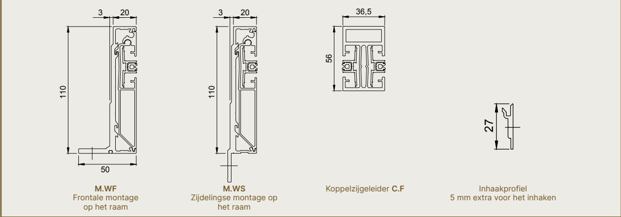
Montage zonder uitvulling
