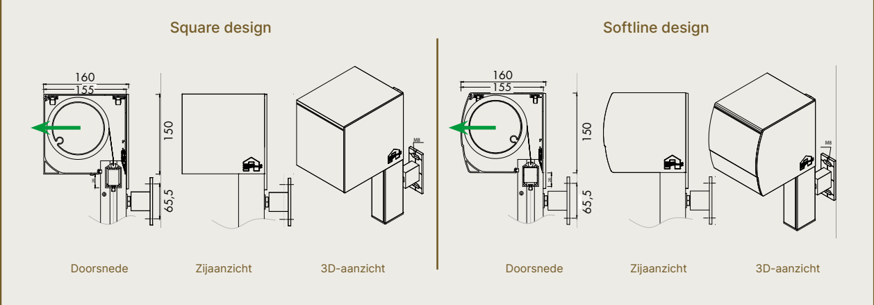
Fixscreen® 100 - Onderlat
