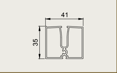
Onderlat
