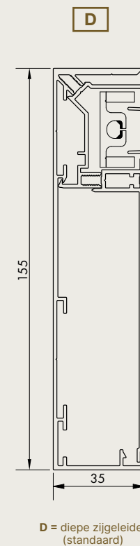
Zijgeleiders
