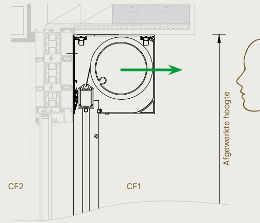
Fixscreen® 150 - Voorbouwtekening binnentoepassing
