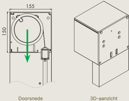
Fixscreen® 150 - MS 7A - Kast
